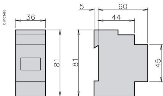
iEM2100/iEM2105 dimensions
