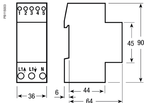
iEM2110/iEM2135/iEM2150/iEM2155 dimensions
